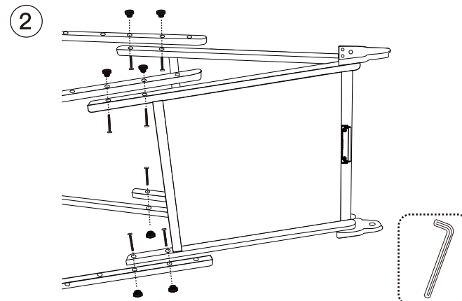
03 Patas de caballete*4 12 Tornillos B*8 13 Tuercas rojas*8
