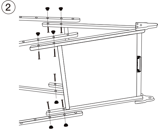
03 Pieds de chevalet*4 12 Vis B*8 13 Écrous rouges*8
